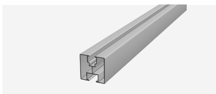
PV-Schiene 40×40 mm M10 Nut unten, M8 Nut oben
