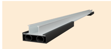
Aluschiene + EPDM Gummi (2x)
