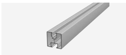
PV-Schiene 40×40 mm M10 Nut unten, M8 Nut oben
