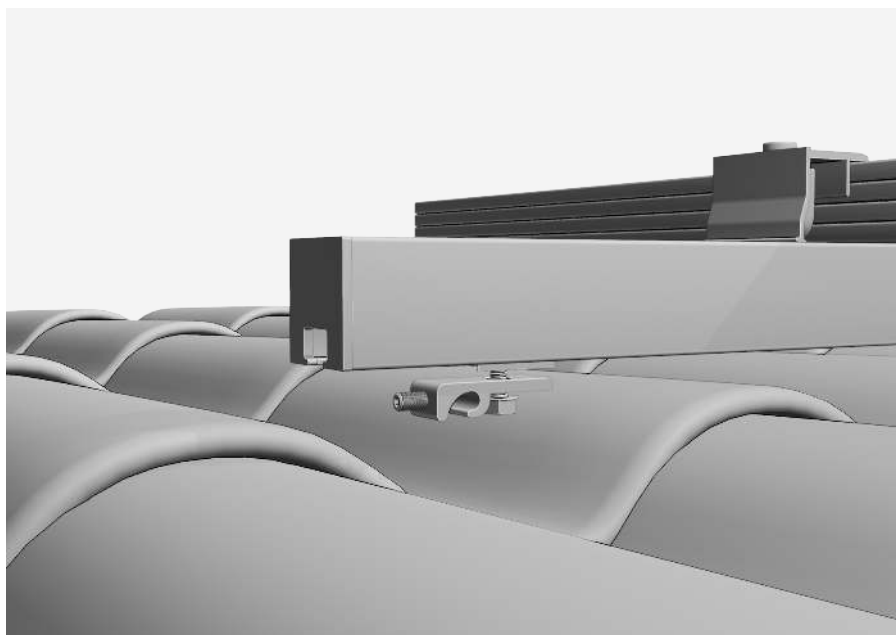
Erdungsklemme
