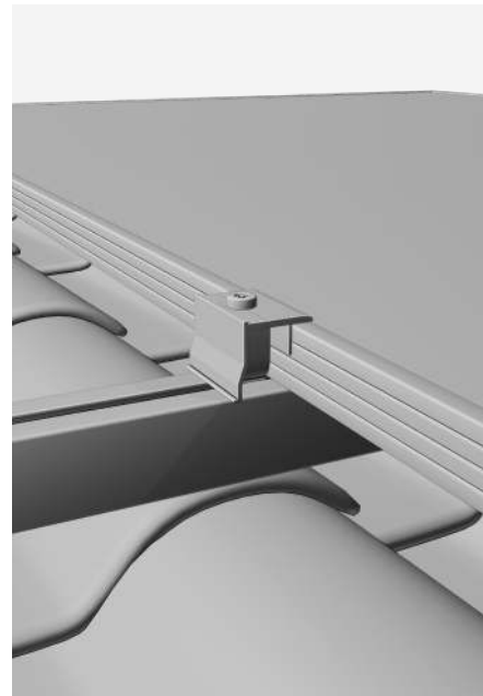
Endklemmen Video
