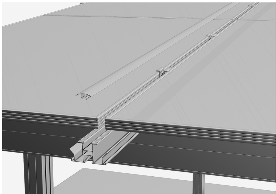
Klemmleiste (lange Moduleseite) 4x 3,00m 4x 2,40m
