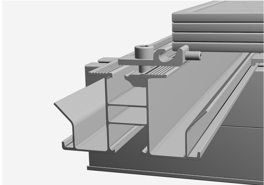
6x Erdungsklemme
