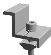
12x Modulklemme (Ende)
