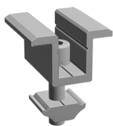
24x Modulklemme (Mitte)
