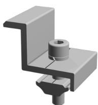
12x Modulklemme (Ende)
