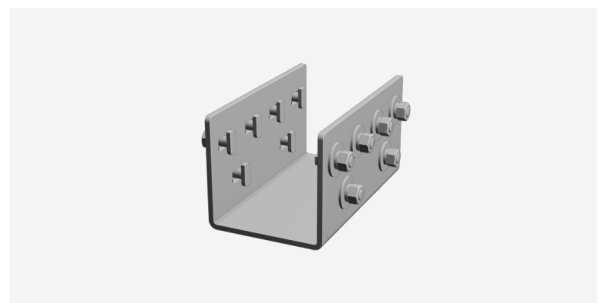
4x Schienenverbinder (L051 mit L051)
