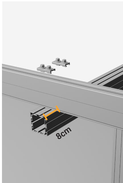
20x Verbinder (R035 auf L051)
